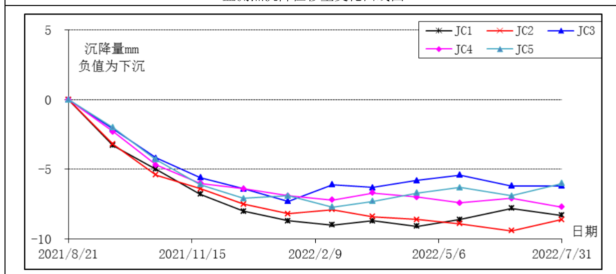
监测点沉降位移量变化曲线图
