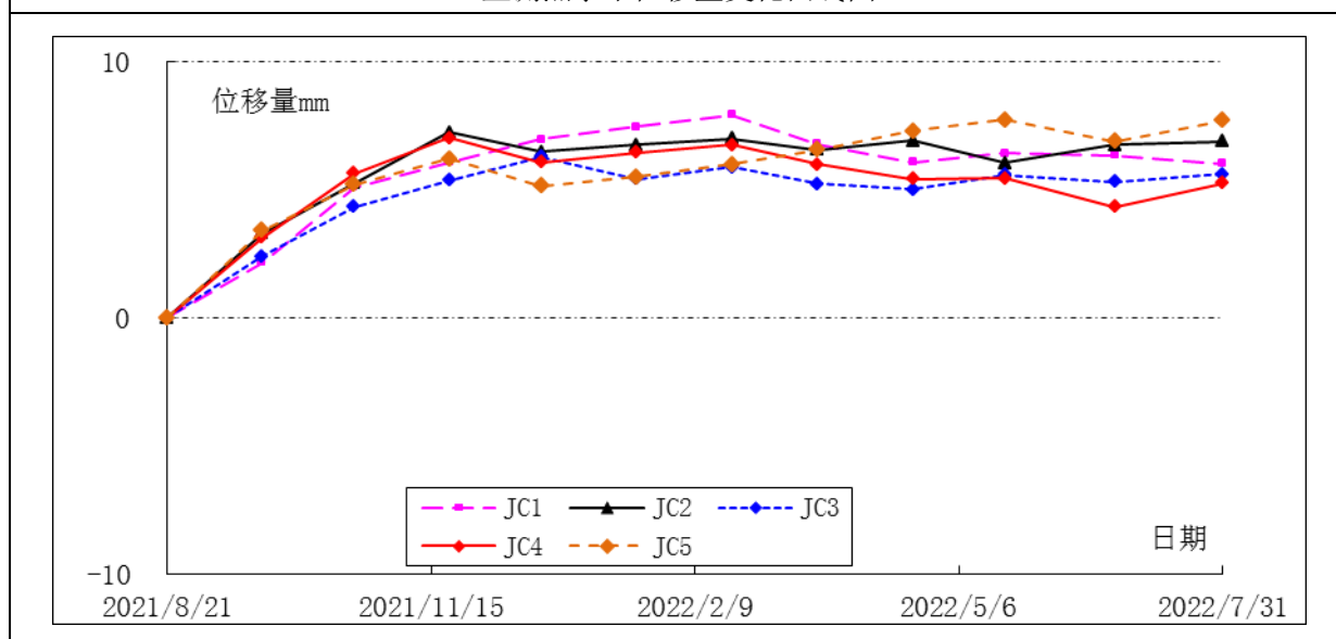
监测点水平位移量变化曲线图
