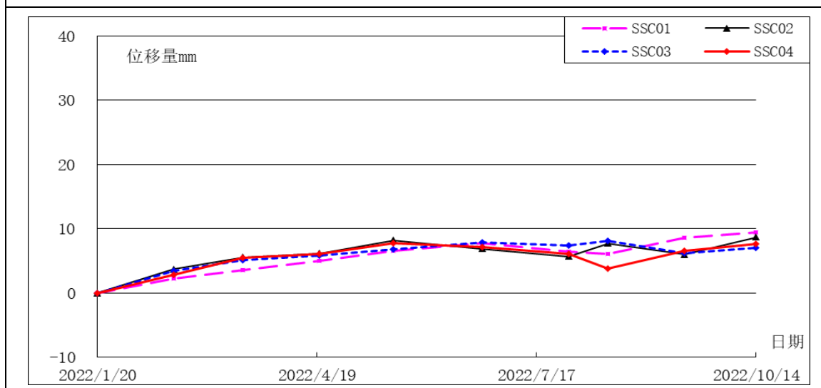
监测点水平位移量变化曲线图
