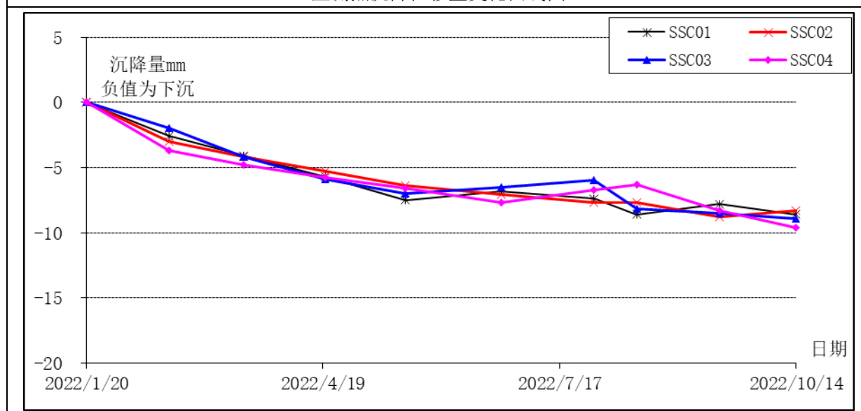
监测点沉降位移量变化曲线图
