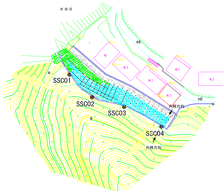
图 1 监测点位置图
